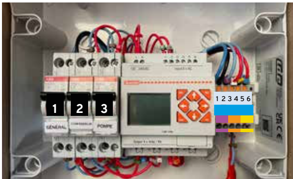
Connexions au tableau électrique.
